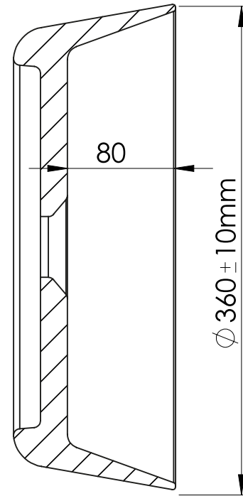
COUPE A-A
